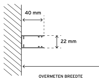
HORIZONTALE DOORSNEDE
